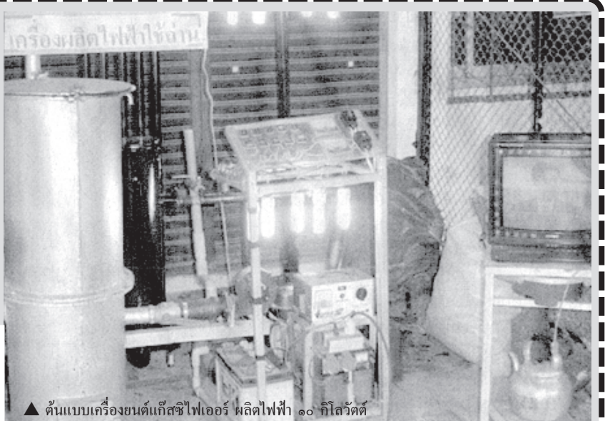
▲ ต้นแบบเครื่องยนต์แก๊สซิไฟเออร์ ผลิตไฟฟ้า ๑๐ กิโลวัตต์
